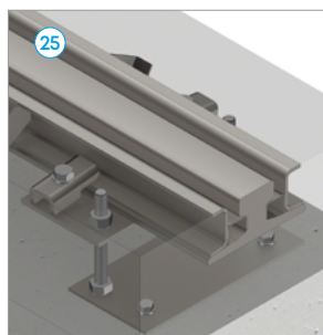
Geleidingsrails
