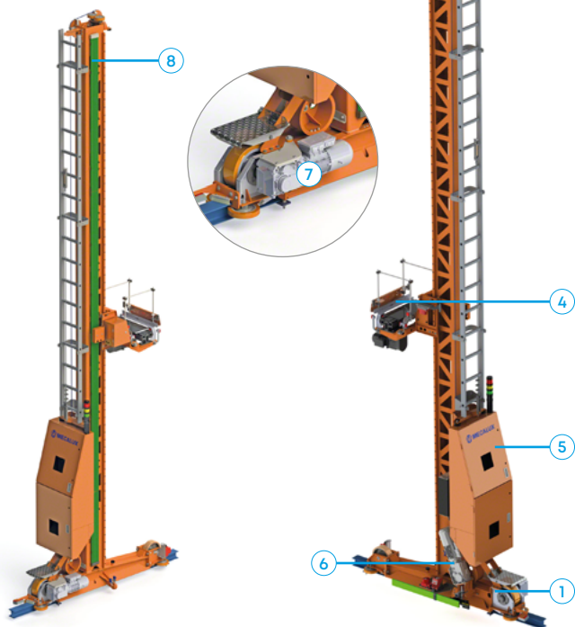
ML50-stapelkraan met enkele mast Verwerkt dozen tot 50 kg op hoogtes tot 9 m.
