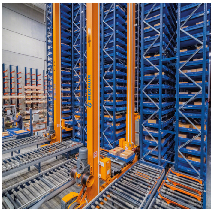
ML100-stapelkraan met enkele mast Bereikt hoogtes tot 12,3 m en transporteert twee dozen van 50 kg.
