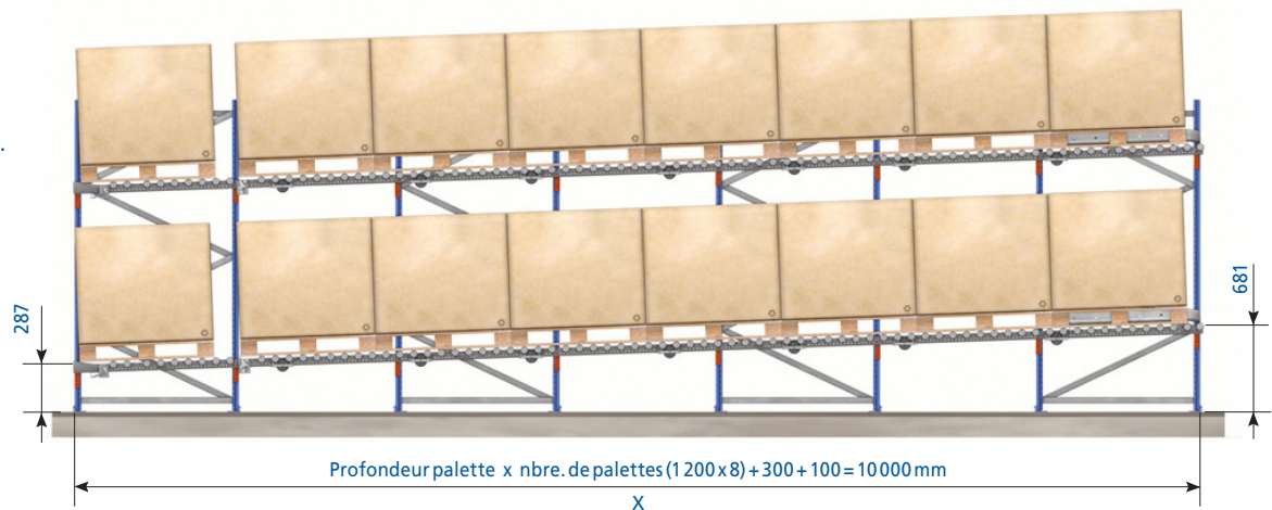
Figure 8. Exemple avec butée de palettes (4 % d'inclinaison).
